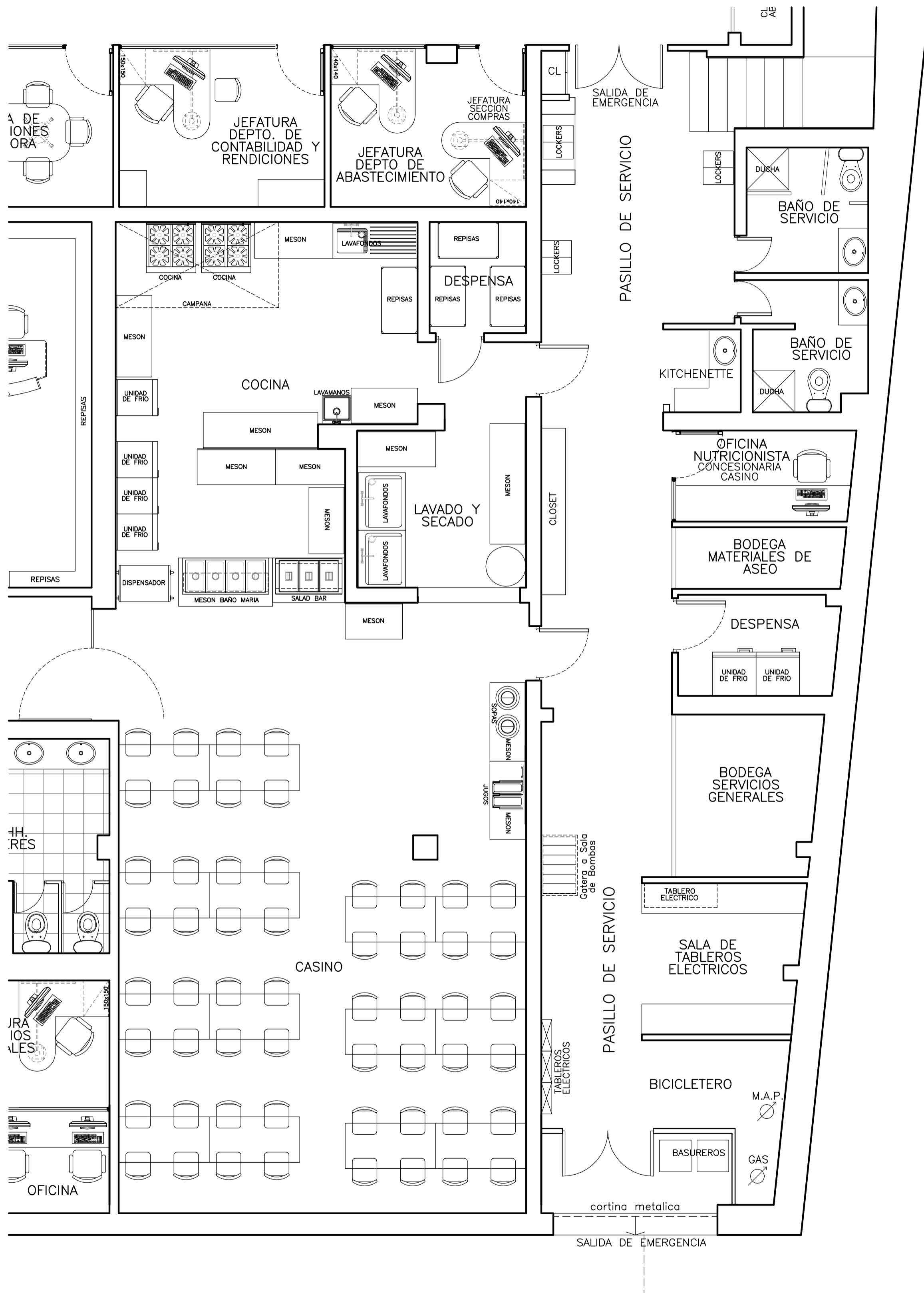
EDIFICIO CASA CENTRAL ALONSO OVALLE N°1180 PLANTA CASINO Escala 1:50
